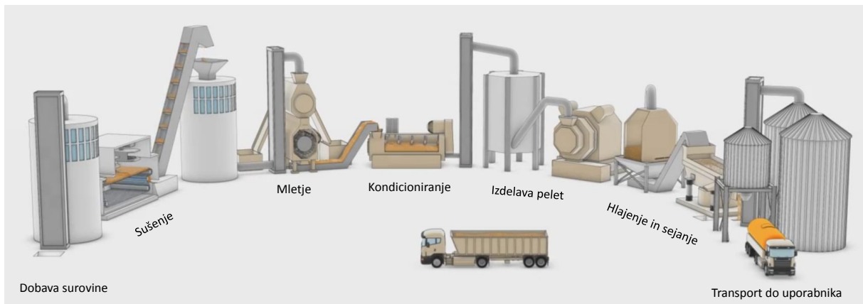
Slika 1: Shema proizvodnega procesa pelet (Vir: EnergieAgentur.NRW)
