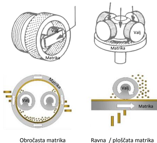
Slika 4: Način proizvodnja pelet z obročasto ali ploščato matriko
